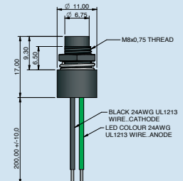
QRM-NV Wires
